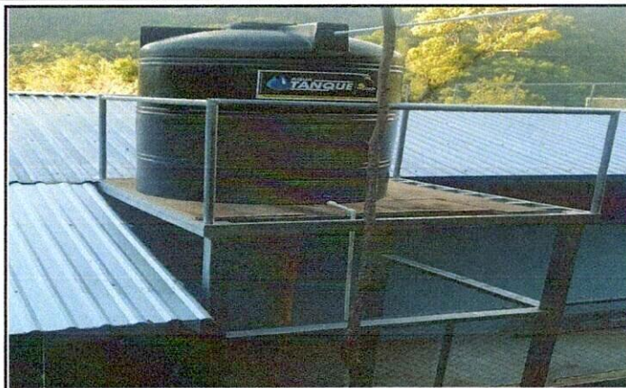
Foto 2: Instalación de torre de metal para el tinaco, tubería para el agua y accesorios.
